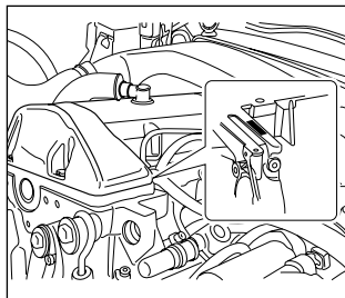
엔진타각번호 (디젤)
