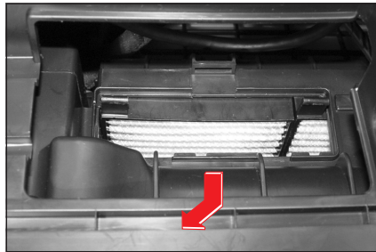
5. 첫번째 에어컨 필터를 아래로 내려 앞으로 탈거합니다.
