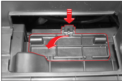
4. 에어컨 필터 커버를 탈거합니다.
