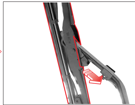
3. 와이퍼 블레이드를 아래로 밀면서 와이퍼 암에서 빼내십시오.
